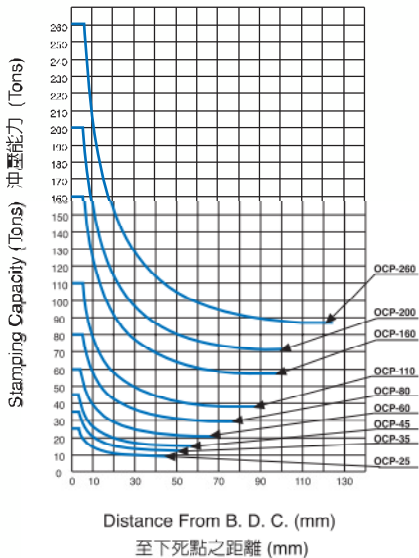
Stroke-Capacity Diagram ( L ) 行程-能力曲線圖 ( L )
