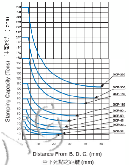
Stroke-Capacity Diagram ( H ) 行程-能力曲線圖 ( H )
